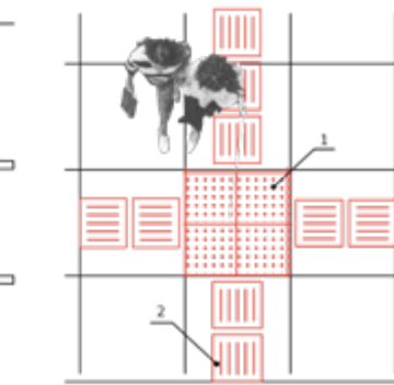
Рисунок 36 — Застосування інформаційної ТС для відображення повороту (розходження): 1 - інформаційна ТС, яка вказує на місце розходження; 2 - направляюча ТС
